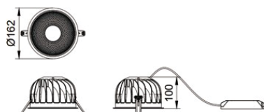
D150 Cut-out range Ø150–155mm
