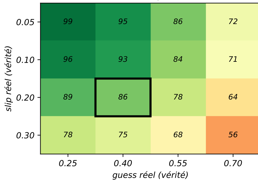
KST adaptatif
