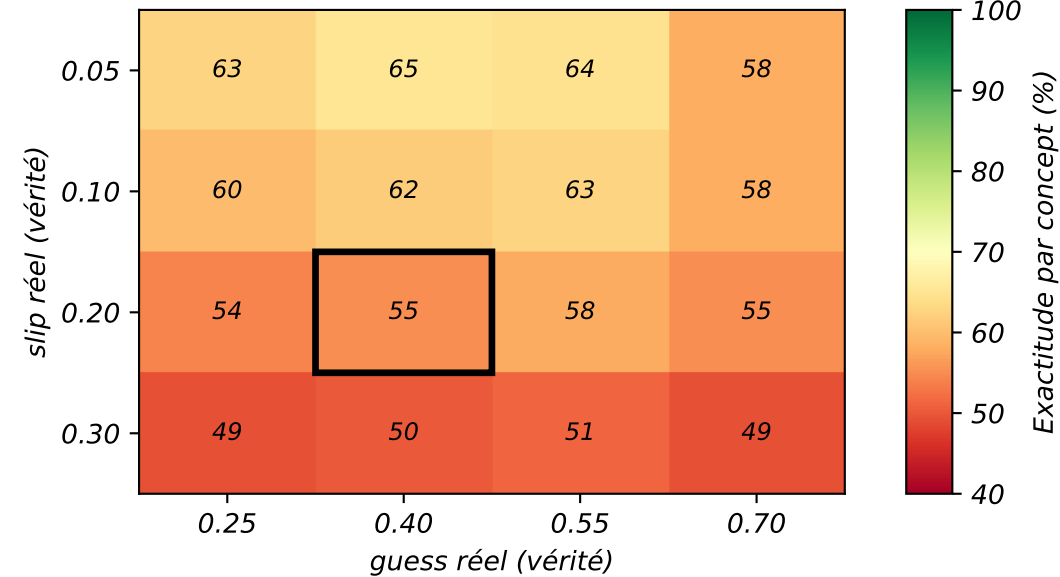
CAT-IRT
