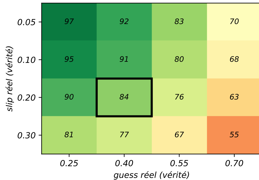
Aléatoire
