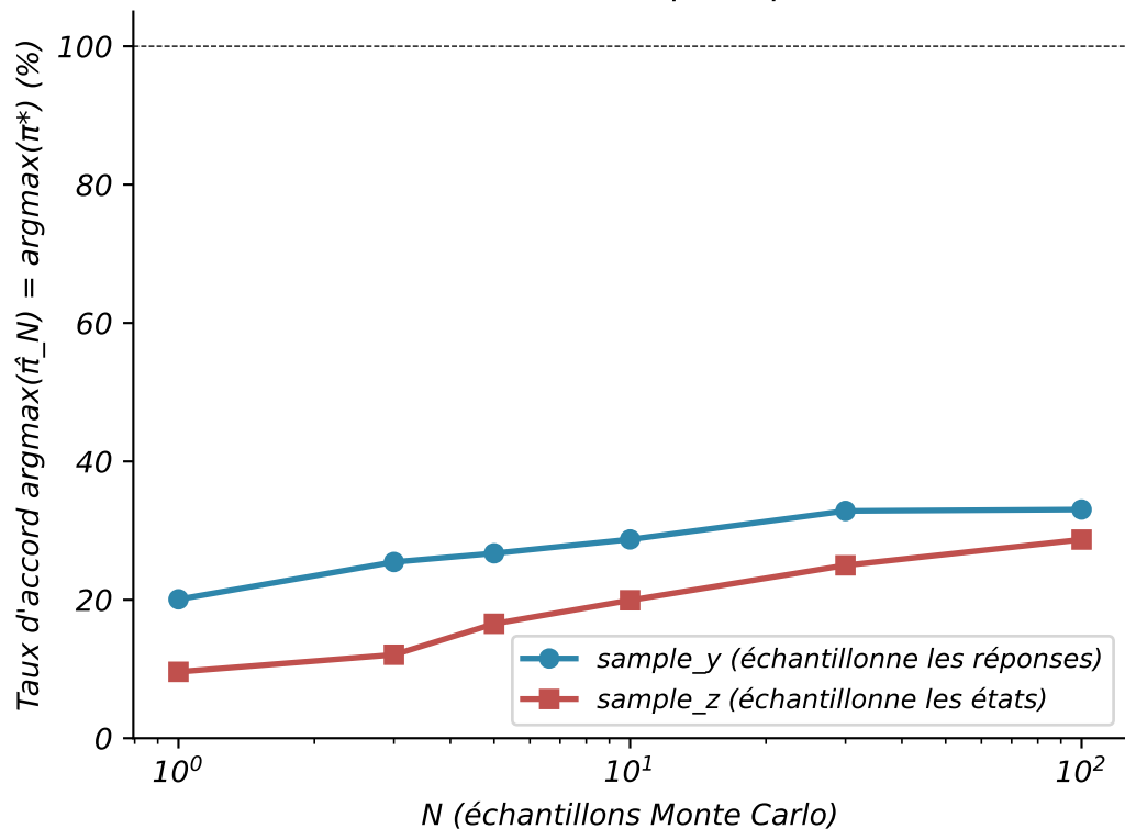
Fidélité de la politique
