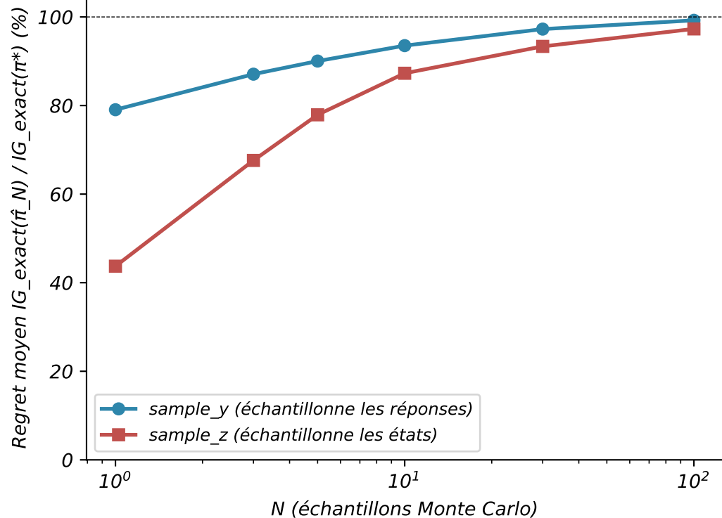
Regret en gain d'information (métrique honnête — cf. plan_action_code.md 1.2)
