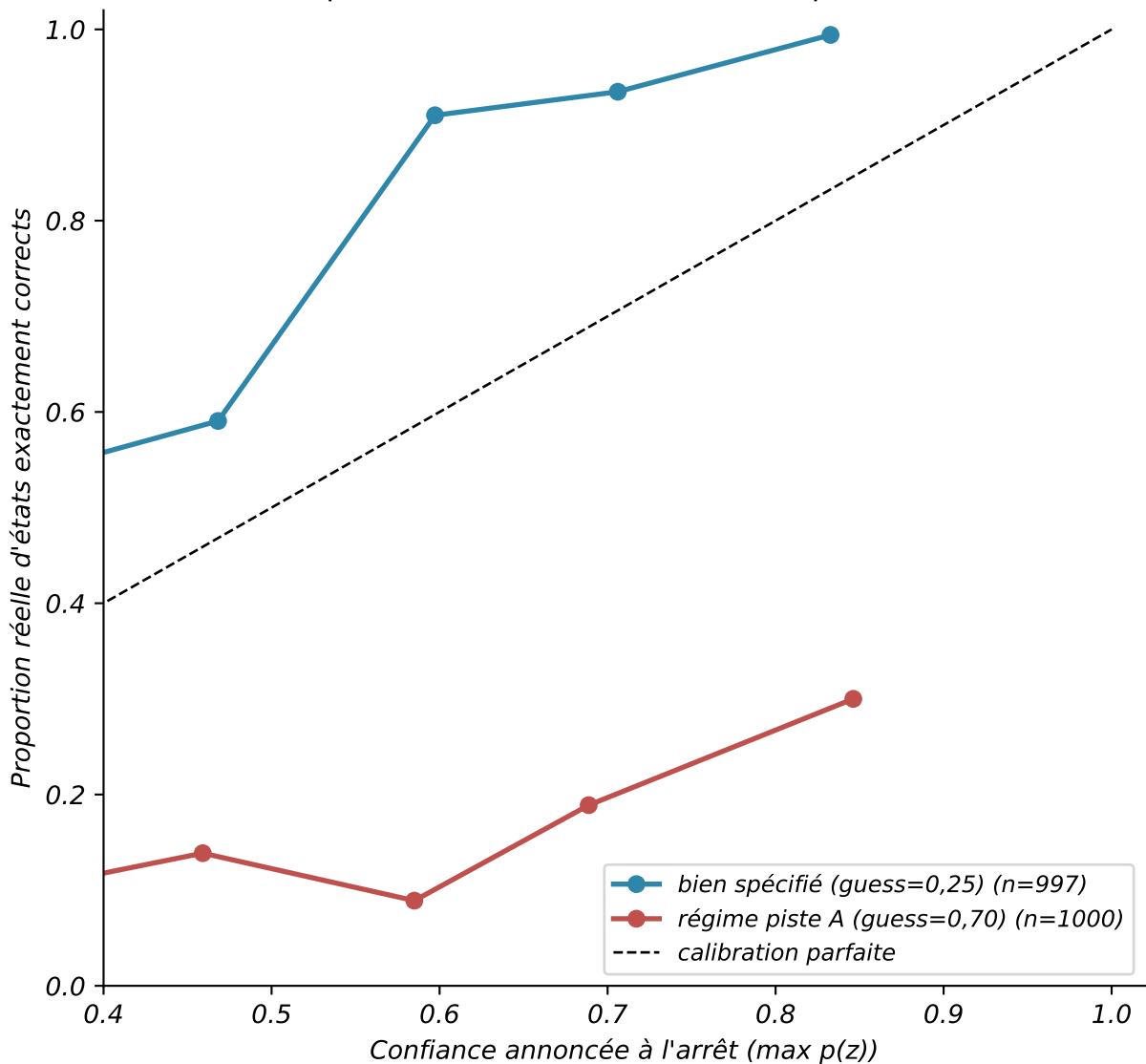
Lot 3.5 — diagramme de fiabilité (politique KST adaptative) sous mauvaise spécification, "90% sûr" ne veut plus dire "9 fois sur 10"
