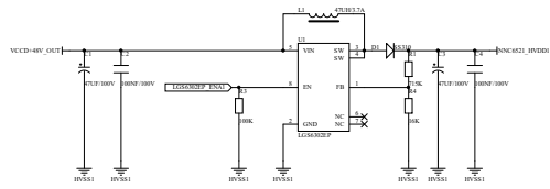
54V升压电源单元
