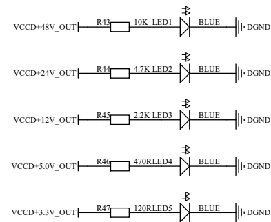
电源指示灯
