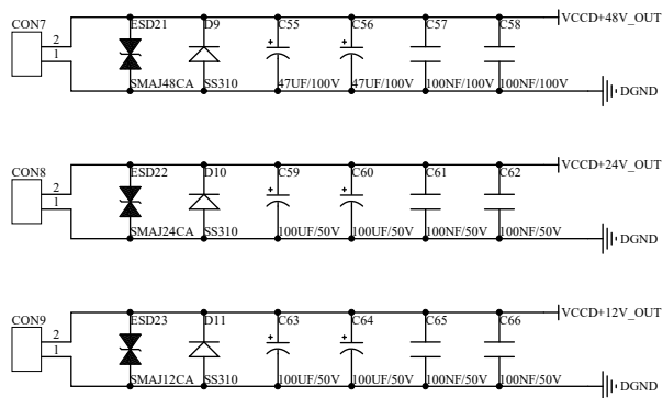
主控板供电输入
