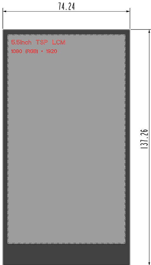
LCD
