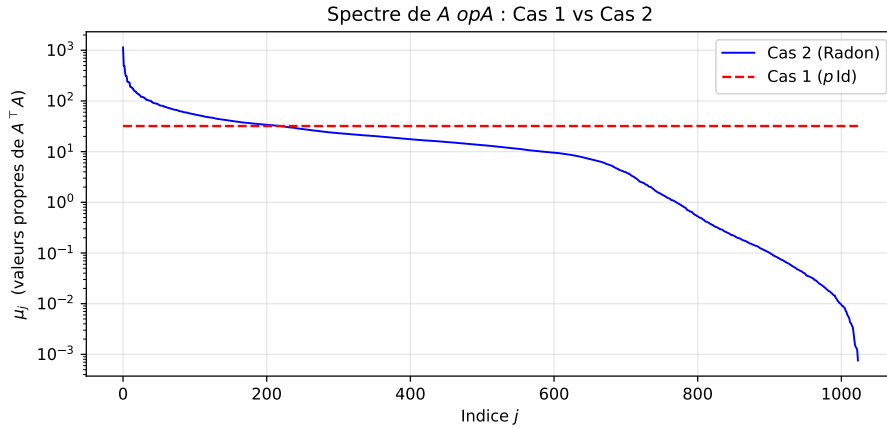
FIGURE 6 – Valeurs propres triées de A^\top A en Cas 2 (Radon, courbe bleue) et en Cas 1 (tirets rouges, \mu_j = p = 32 constant). L'axe vertical est logarithmique.
