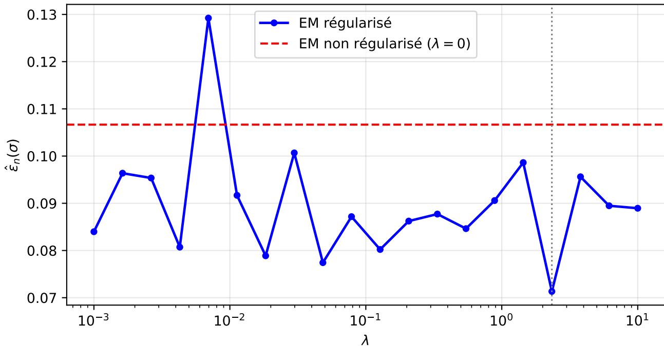
Erreur en fonction de \lambda ( n = 50, \sigma = 0.3, M = 20 )
