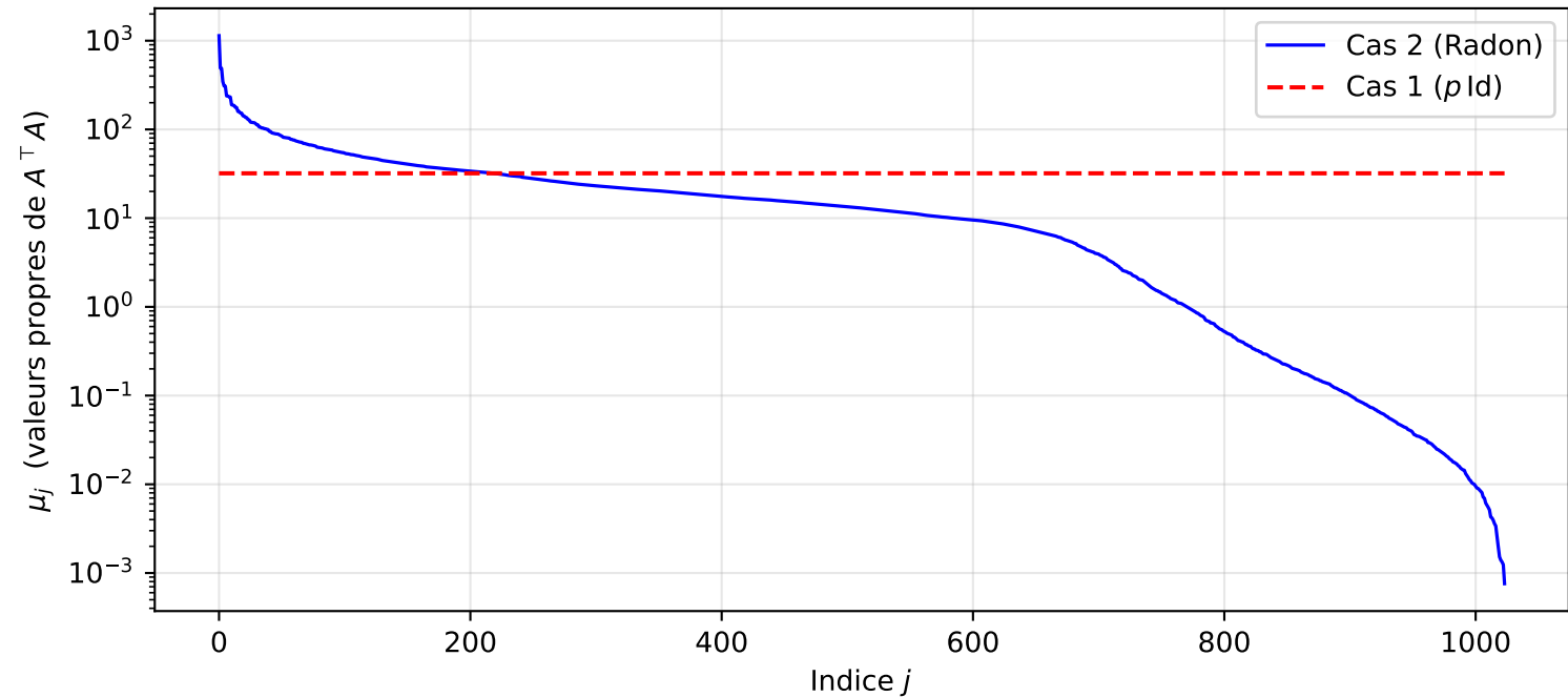
Spectre de A_{opA} : Cas 1 vs Cas 2
