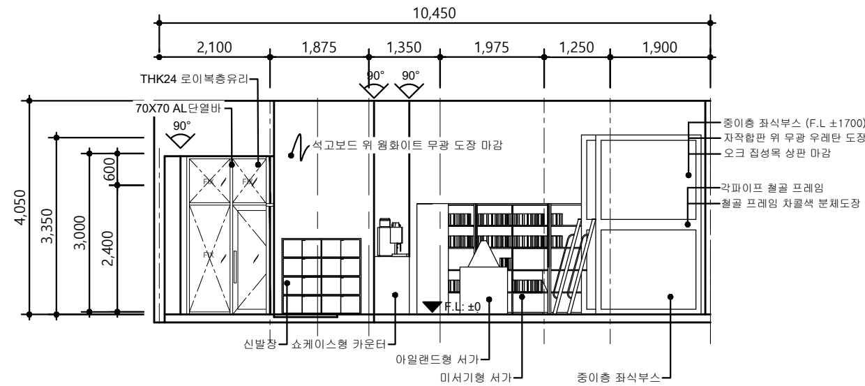
내부입면도-B
