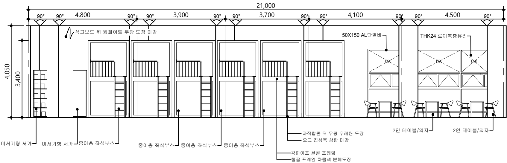
내부입면도-C
