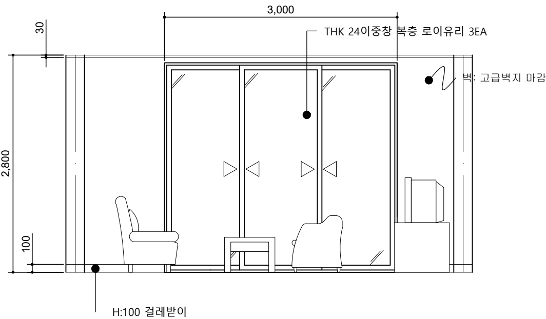
내부입면도 b
