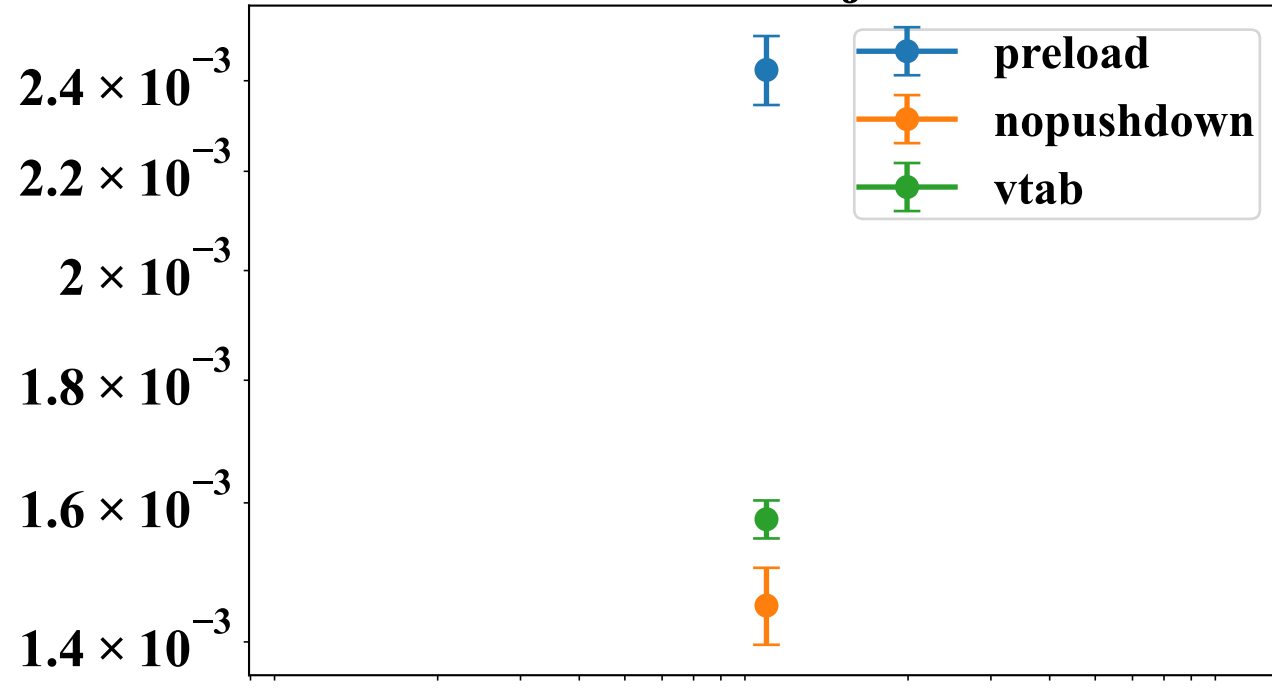
locProj
