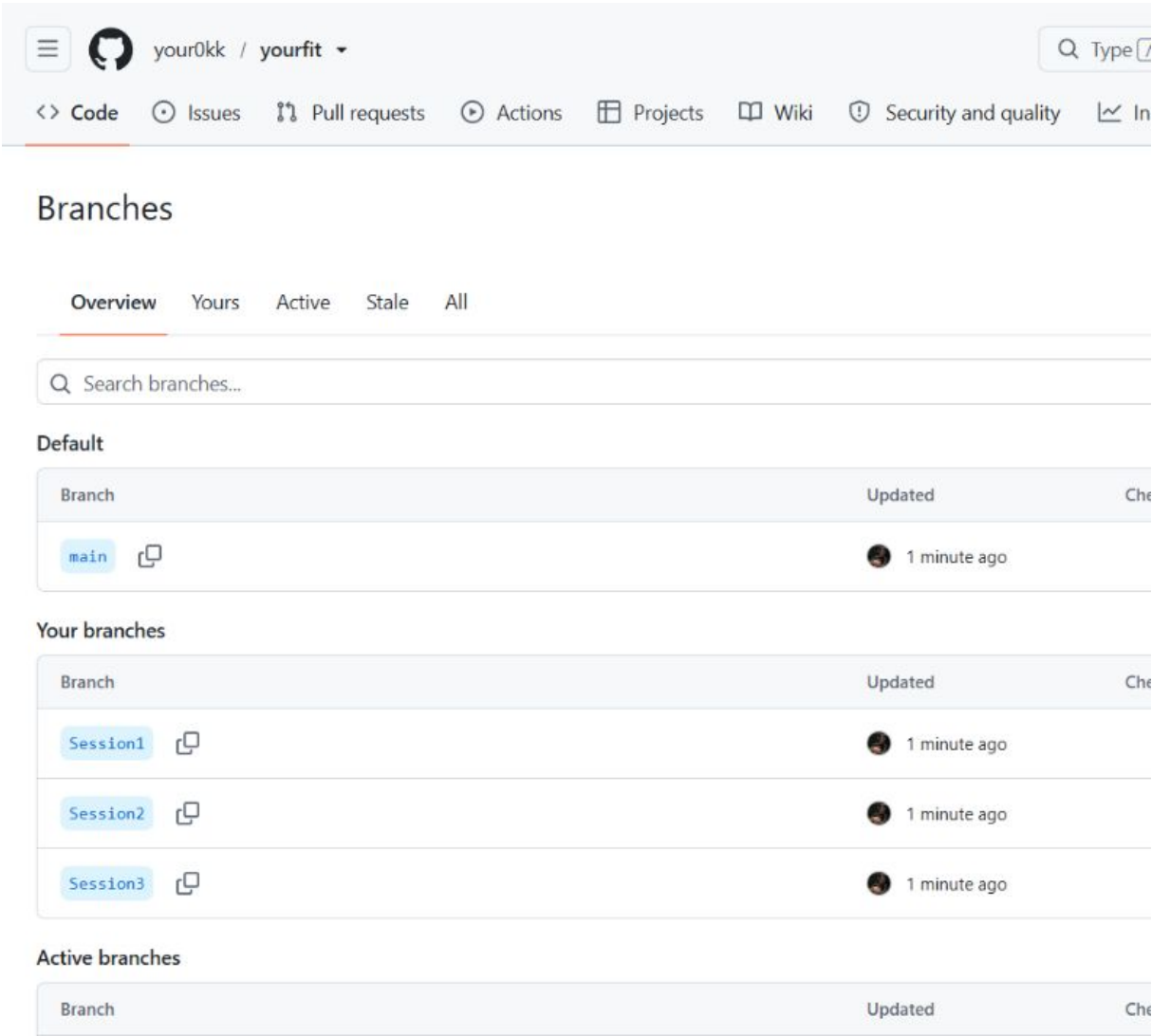
Рисунок 1 Список веток репозитория yourfit
