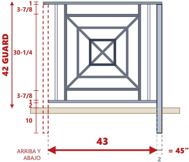
LARGO DE LA SECCIÓN 45" (3'-9")
