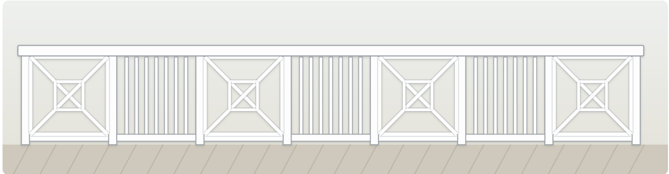
Vista de presentación — sección con el motivo alternando con sección de piques · top cap continuo · Color y medidas finales según shop drawing.
