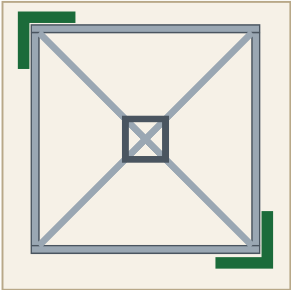
TOPES "L" EN 2 ESQUINAS OPUESTAS (45°) 1) marco C · 2) D1 · 3) D2+D2 · 4) cuadrito E
