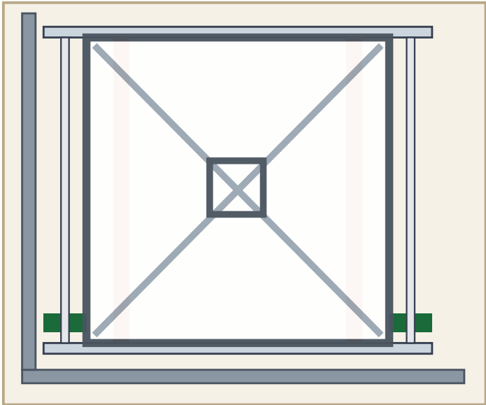
BLOQUES 2" · RIELES CONTRA GUÍA Y SEPARADORES 35-1/2" EL CUADRO TERMINADO CAE ENTRE LOS RIELES Y SE PUNTEA
