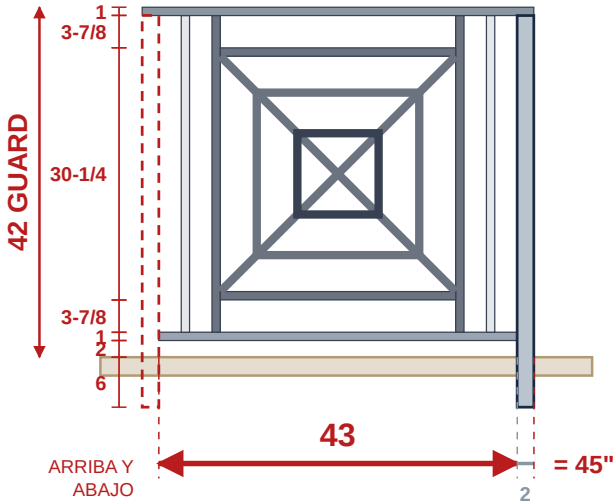
LARGO DE LA SECCIÓN 45" (3'-9")
