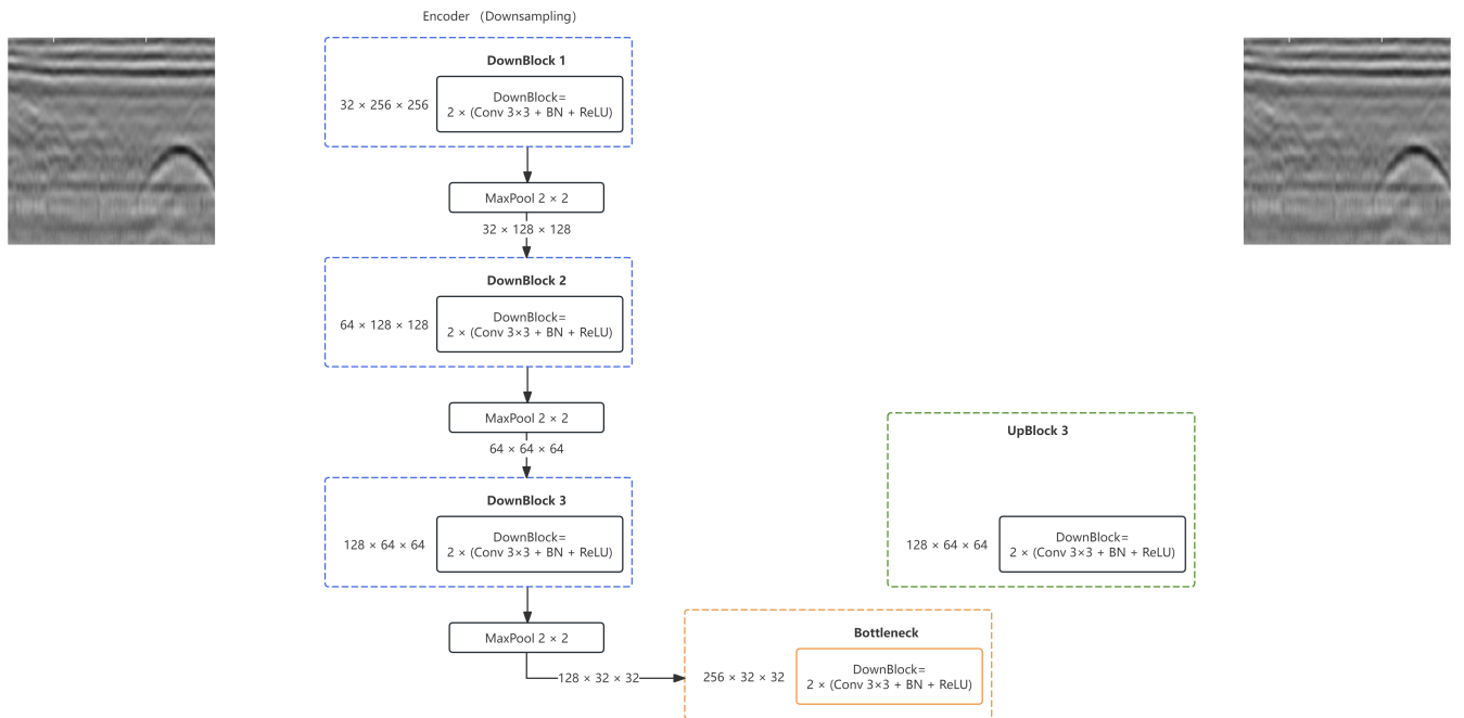
Fig. 3. unet
