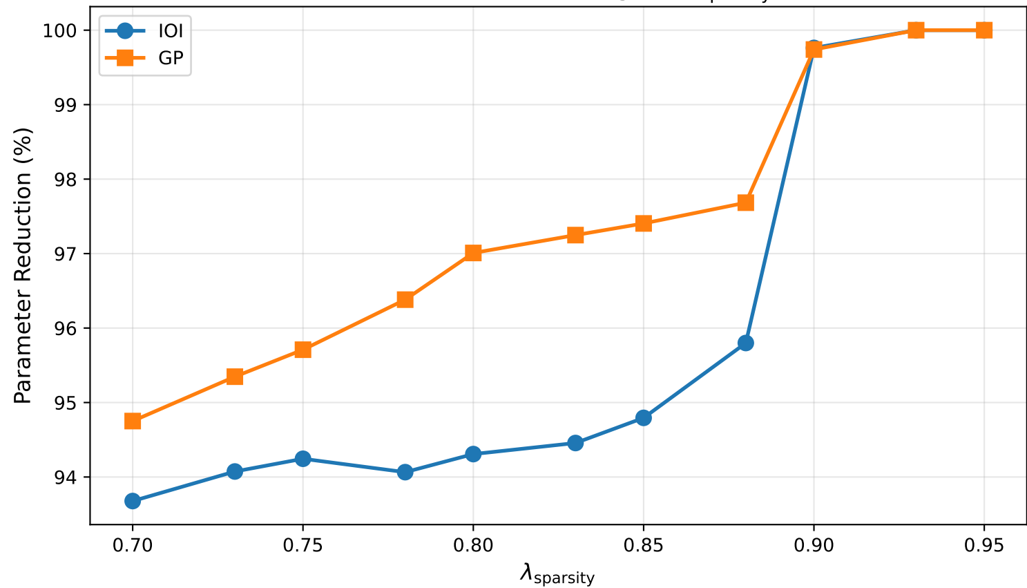
Llama-3.1-8B: Pruning vs. \lambda_{\text{sparsity}}
