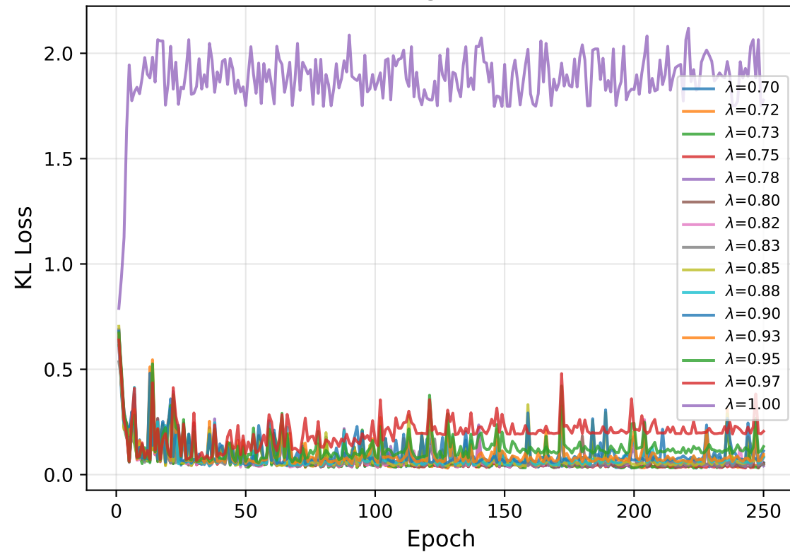
KL Divergence Loss
