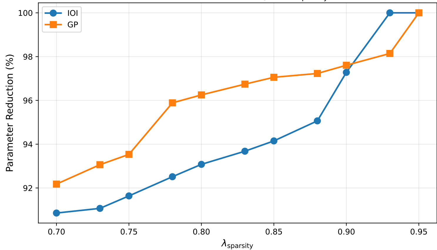
Llama-3.2-1B: Pruning vs. \lambda_{\text{sparcity}}
