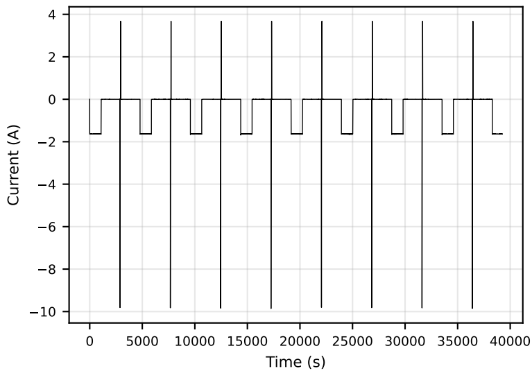
HPPC
