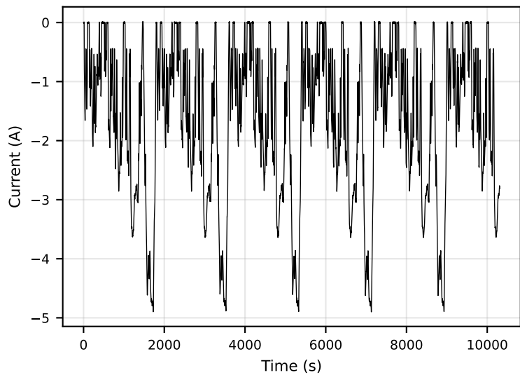
WLTC
