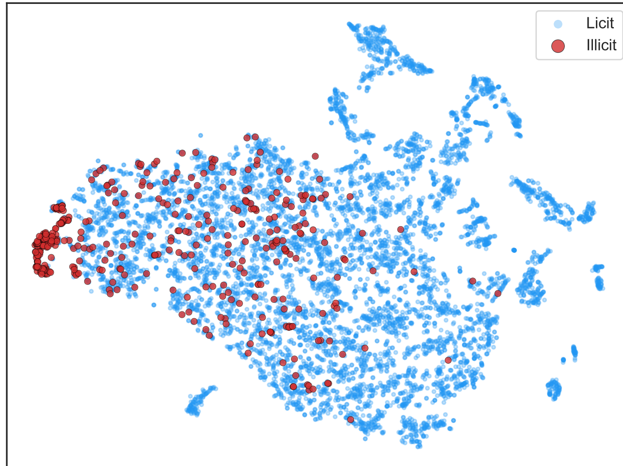
M3: R-GCN+Hetero (AUC=0.8678)
