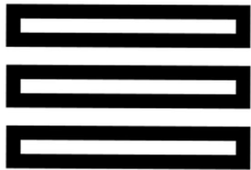
건(乾)_하늘
