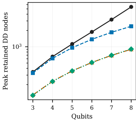
GHZ
