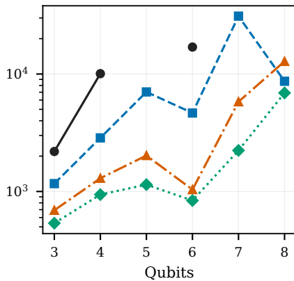
Clifford+T
