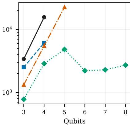
QFT
