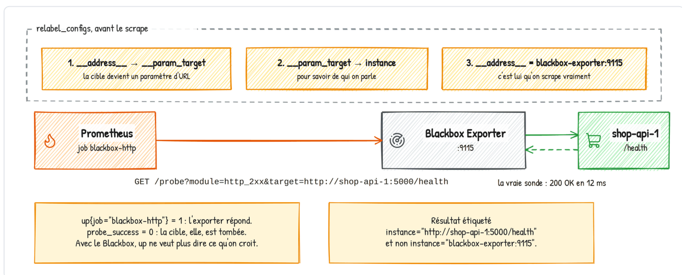
Le chemin d'une sonde Blackbox
