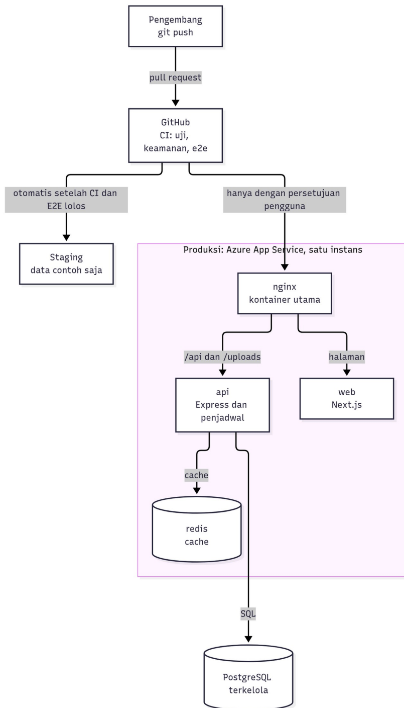
Gambar: Penempatan — dari kode sampai staging dan produksi
