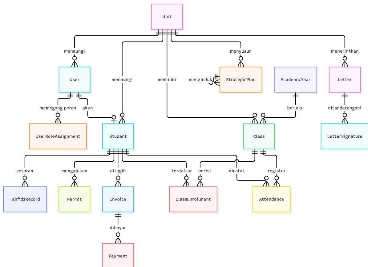
Gambar: Model data tingkat ranah — model Prisma utama dan relasinya
