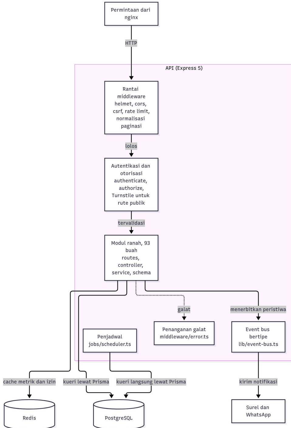
Gambar: C4-3 Komponen — bagian utama di dalam kontainer API
