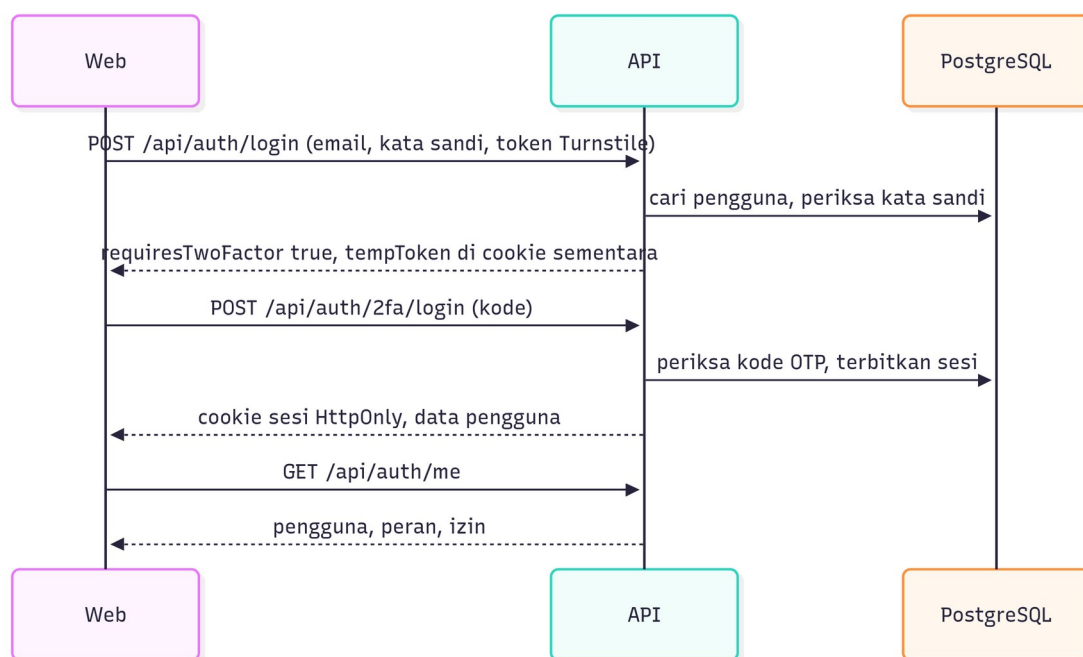
Gambar: Urutan masuk akun admin yang sudah mengaktifkan 2FA
