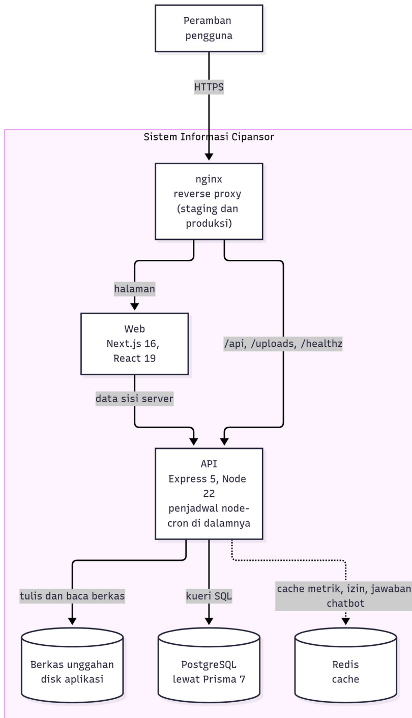
Gambar: C4-2 Kontainer — bagian yang berjalan sendiri dan cara mereka berhubungan
