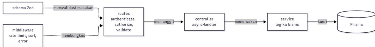
Gambar: Lapisan satu modul API — satu permintaan dari rute sampai basis data
