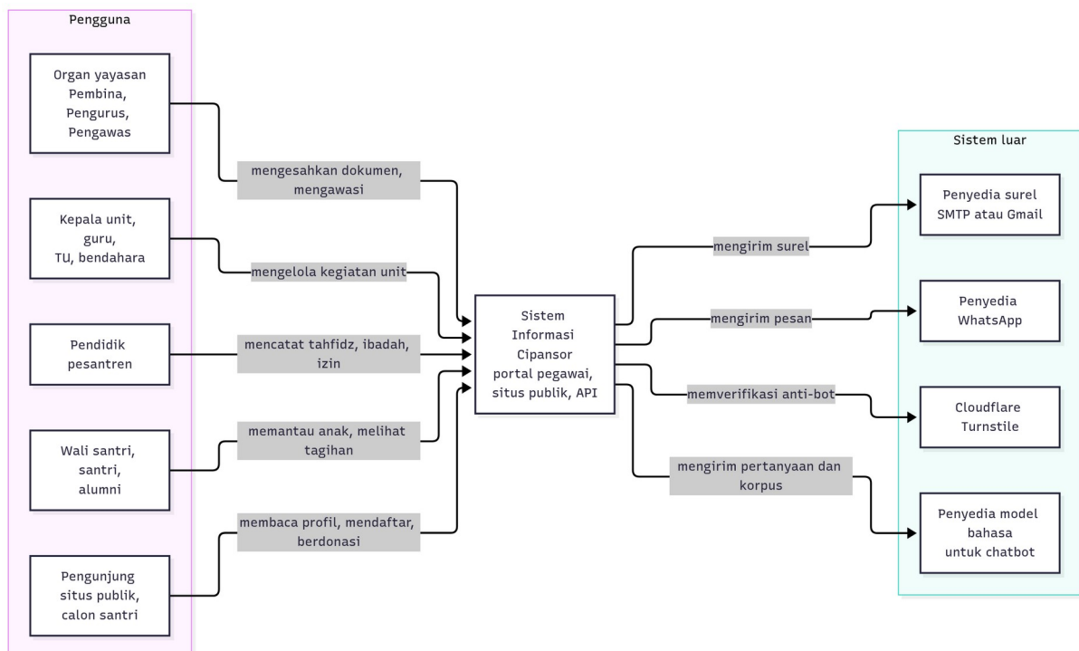
Gambar: C4-1 Konteks — siapa memakai Cipansor dan sistem luar mana yang dipanggilnya
