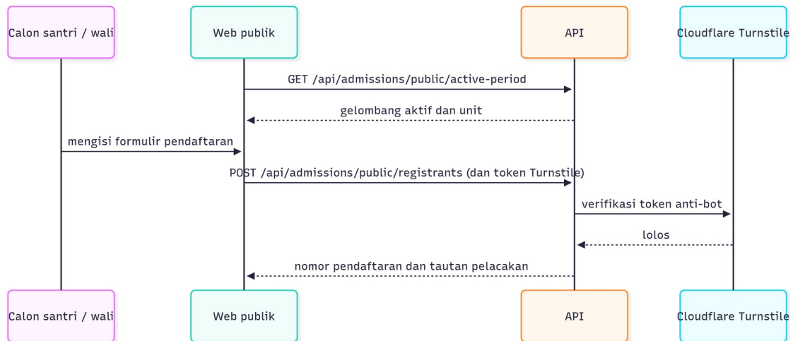
Gambar: Urutan pendaftaran publik pada SPMB
