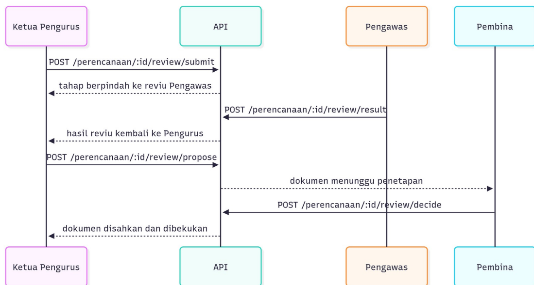
Gambar: Urutan pengesahan dokumen tingkat yayasan
