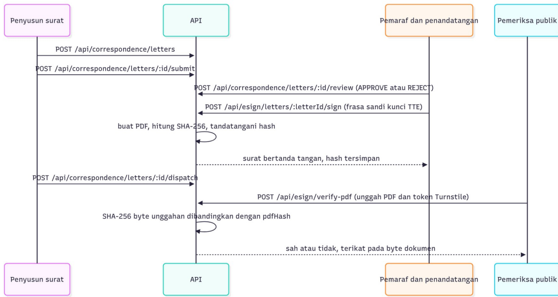
Gambar: Urutan penerbitan naskah dinas dan verifikasi publiknya
