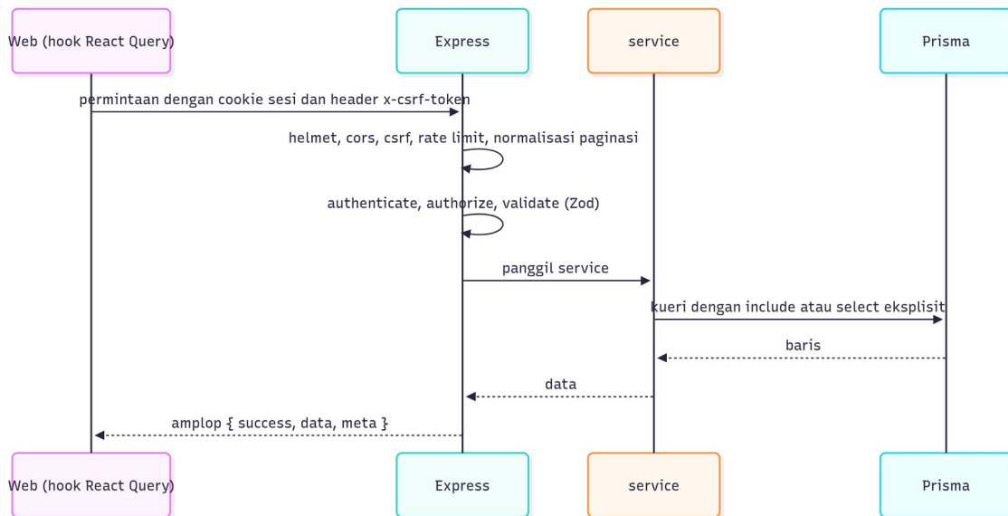
Gambar: Urutan satu permintaan terautentikasi melewati middleware
