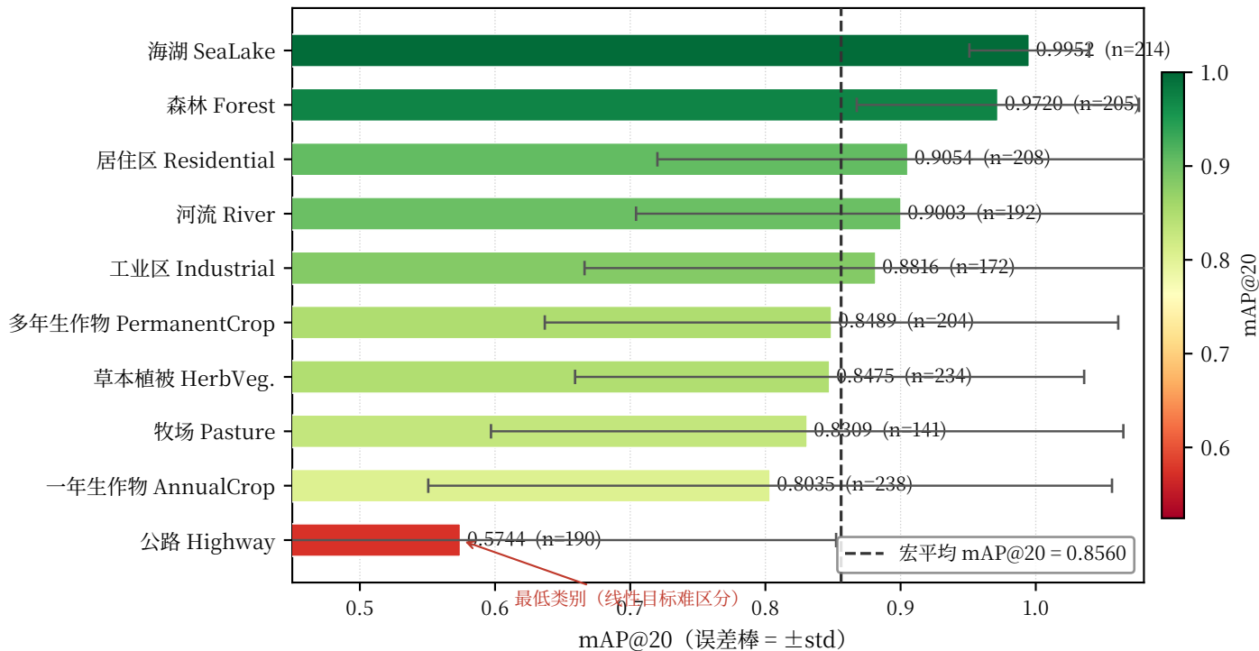
图 5-3 分类检索性能 (mAP@20) — EuroSAT 10 类, 按均值降序排列
