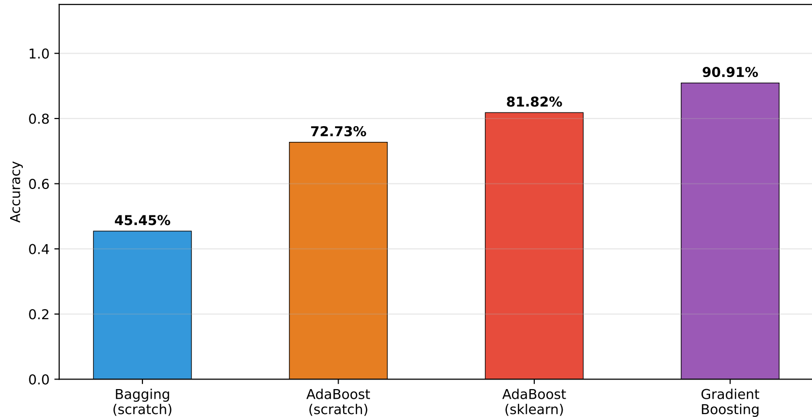
Comparaison des méthodes d'ensemble (Classification binaire)
