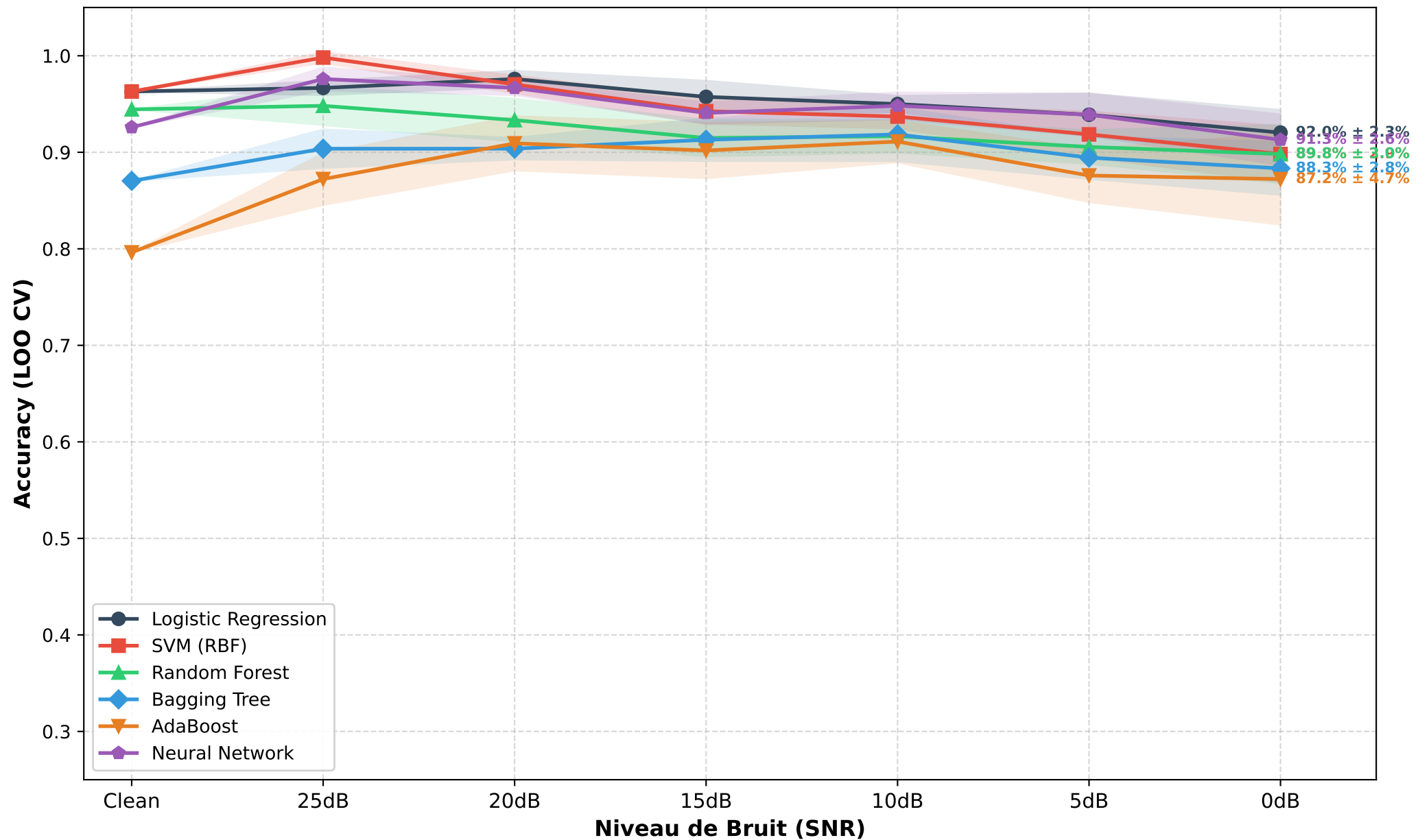
Résilience au Bruit des Classifieurs avec Intervalles de Confiance (MFCC Summary)
