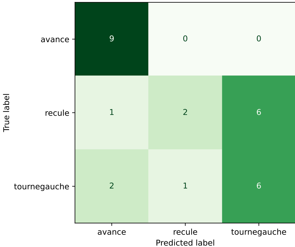
PyTorch — Régression logistique (Acc=62.96%)
