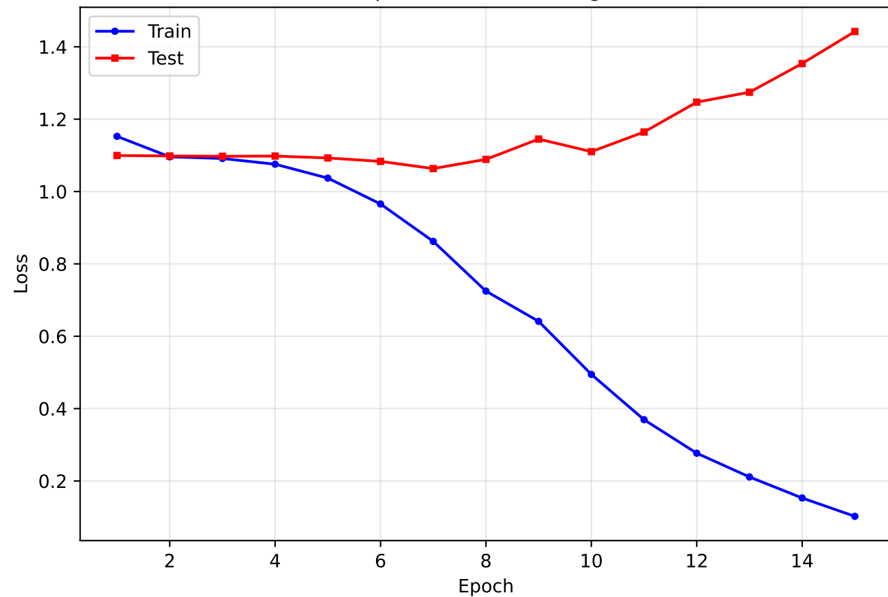
Courbes de perte — CNN 1D (signaux bruts)
