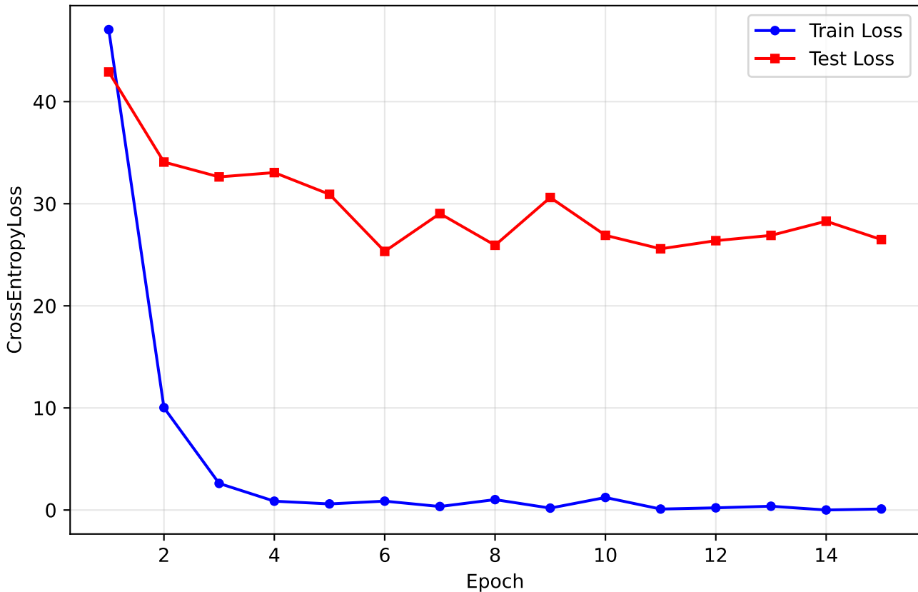
Courbes de perte — Régression logistique (PyTorch)
