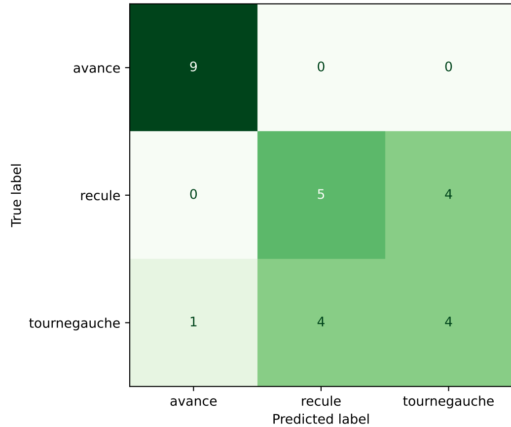
FNN Régularisé (Acc=66.67%)
