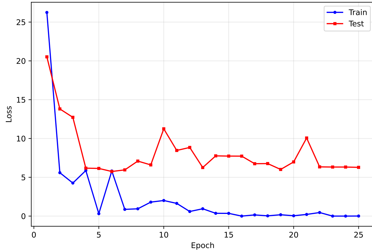
Courbes de perte — FNN Régularisé
