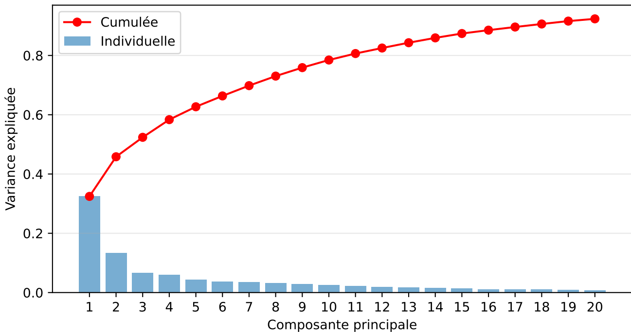
Variance expliquée par l'ACP sur |\hat{X}|
