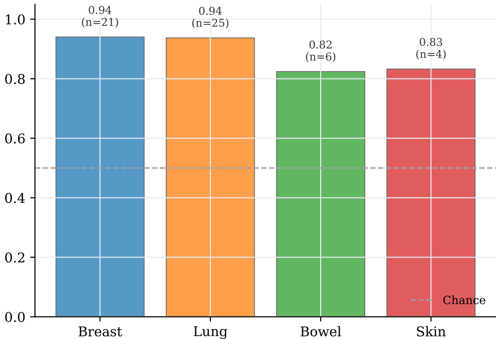
Detector AUROC
