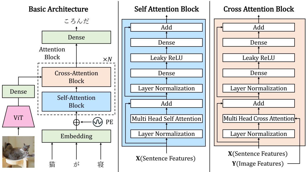
図 2 Warai Transformer (WiT) の構造
