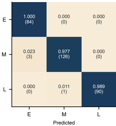
DC-PSR
