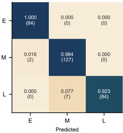
MTF-AViTK
