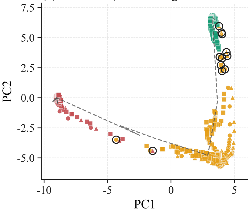
(d) Shared h_{c,t} / true stage
