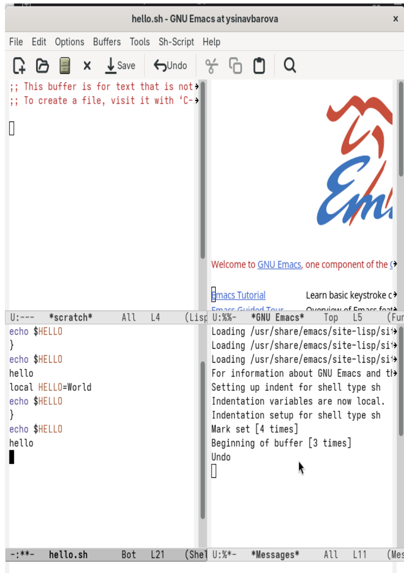
Рисунок 2.11: Четыре буфера
