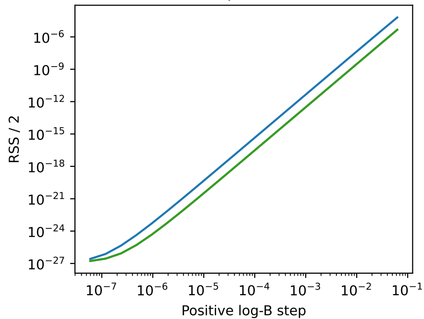
Actual endpoint: atom 10
