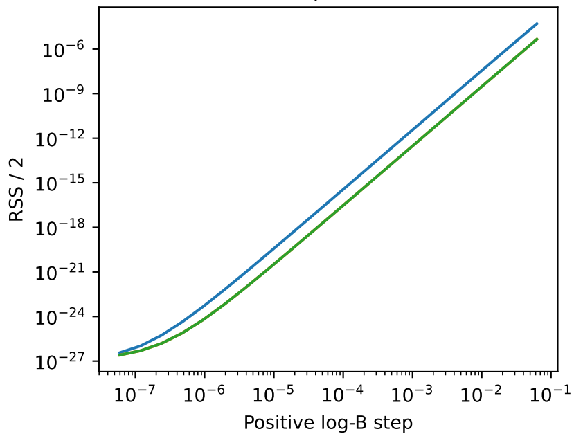
Actual endpoint: atom 6
