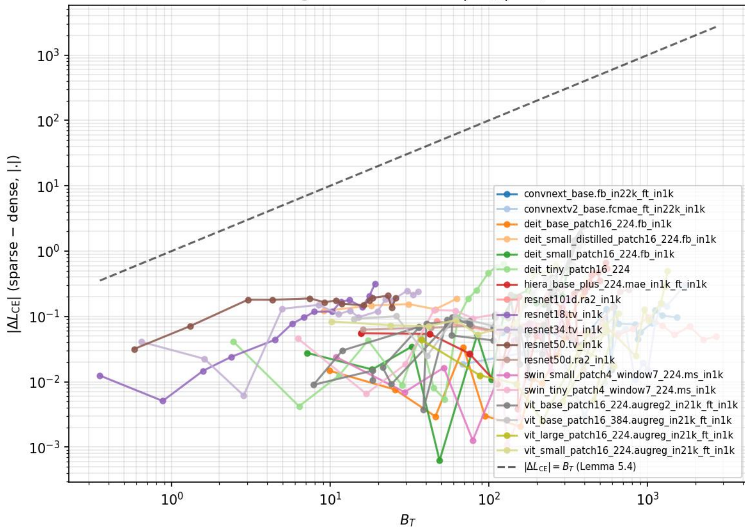
Bridge 2 — Lemma 5.4: |\Delta L_{CE}| \leq B_T
