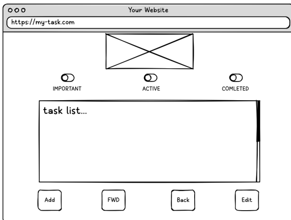
Ekran początkowy
