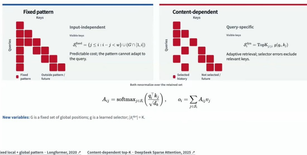
图 16: 稀疏注意力两族：固定模式 S_{\text{fix}} 依赖位置，内容相关 S_{\text{dyn}} 用 TopK 选键 16
