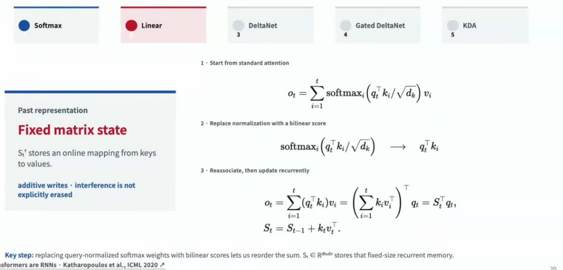
图 12: 线性注意力三步：去掉 softmax 归一化、改用双线性分数、重结合为固定状态 S^{12}
