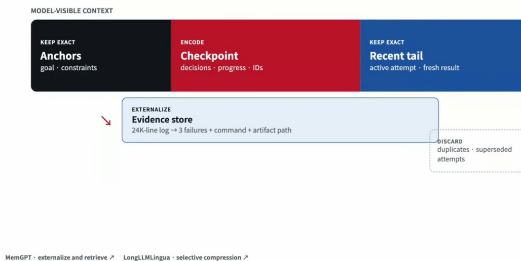
图 37: 压缩中保留什么: 锚点与最近尾部精确保留, 中段编码为 checkpoint, 证据外置到 evidence store 37
