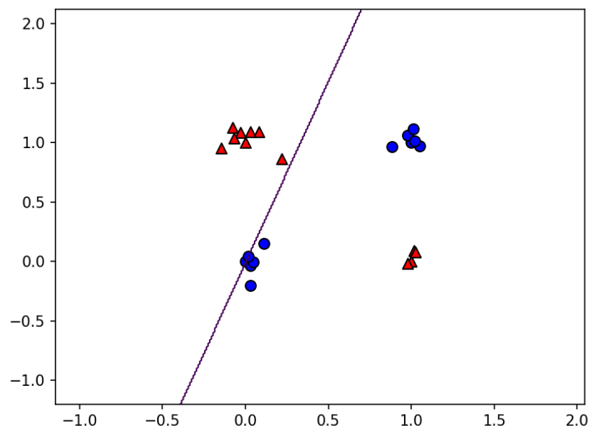
XOR任务
