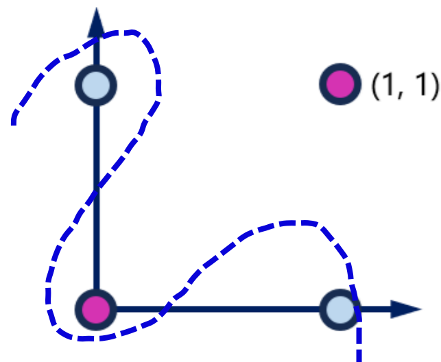
XOR
