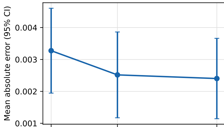
c C_B : hidden-trajectory MAE
