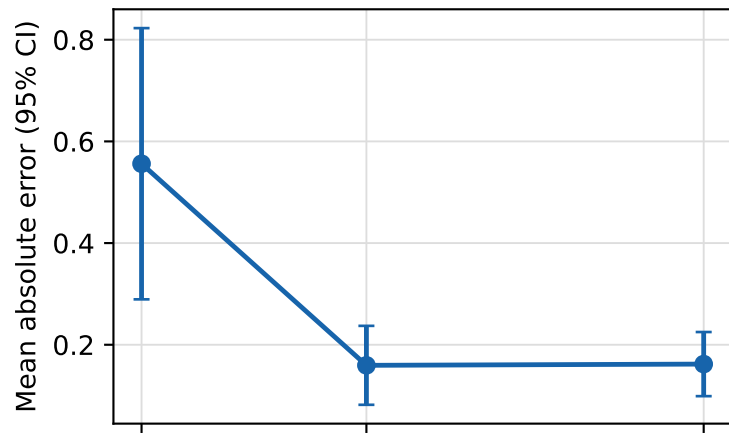
d T : hidden-trajectory MAE
