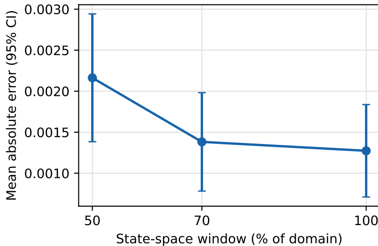
c C_B : hidden-trajectory MAE
