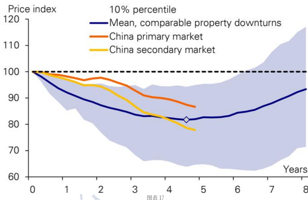
图17：调整的持续时间和深度已与其他经济体的典型住房下行周期相当
