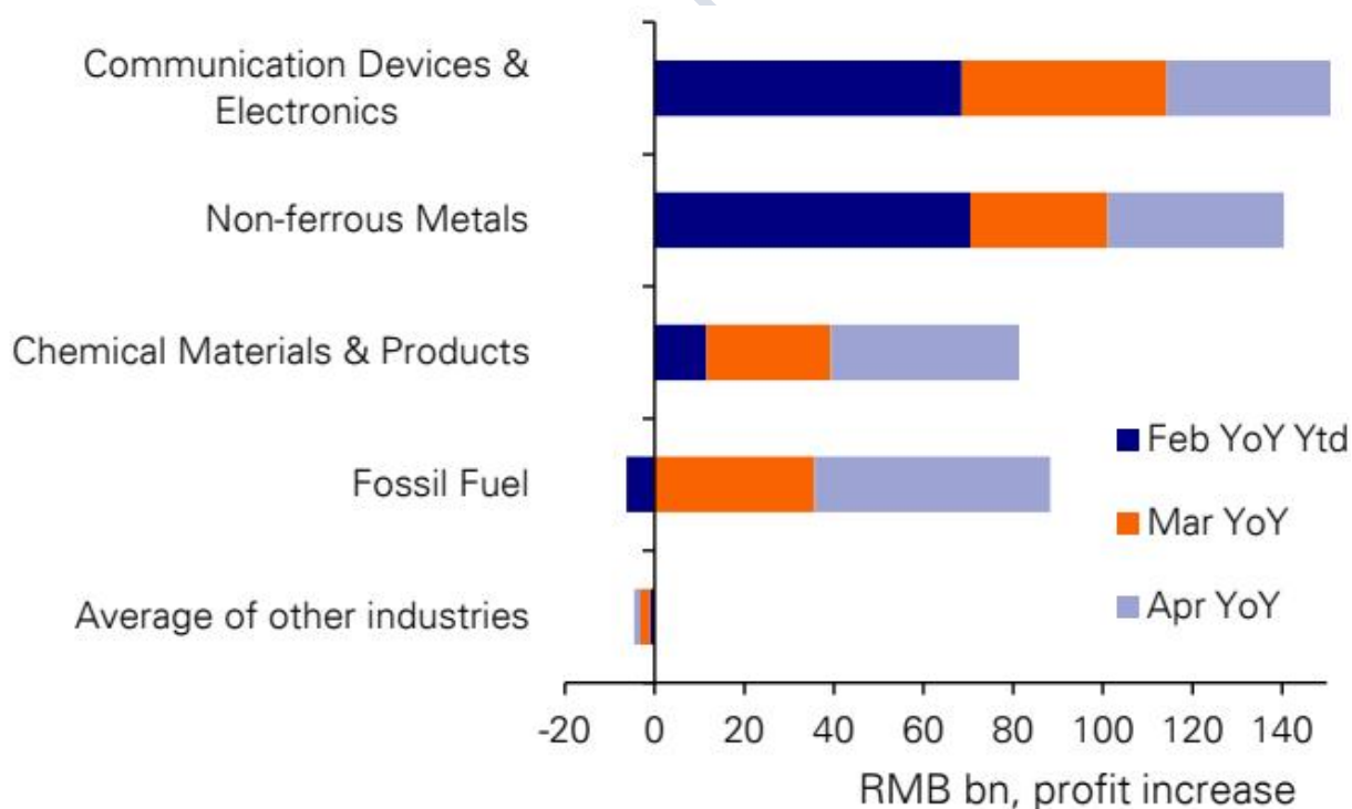
图16：工业企业利润显著改善，尽管集中在少数行业
