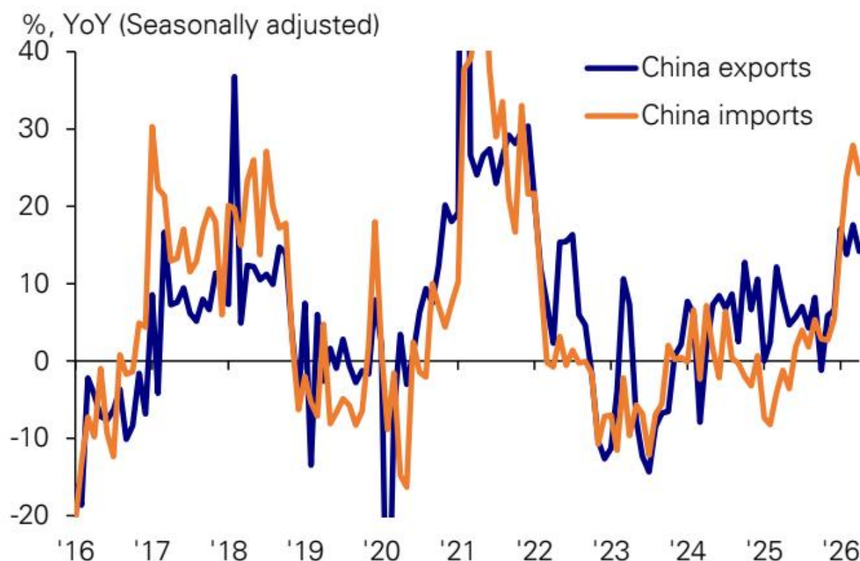
图13：出口和进口增速远超预期
