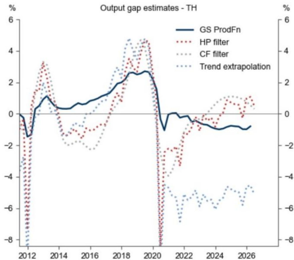
图表 16
