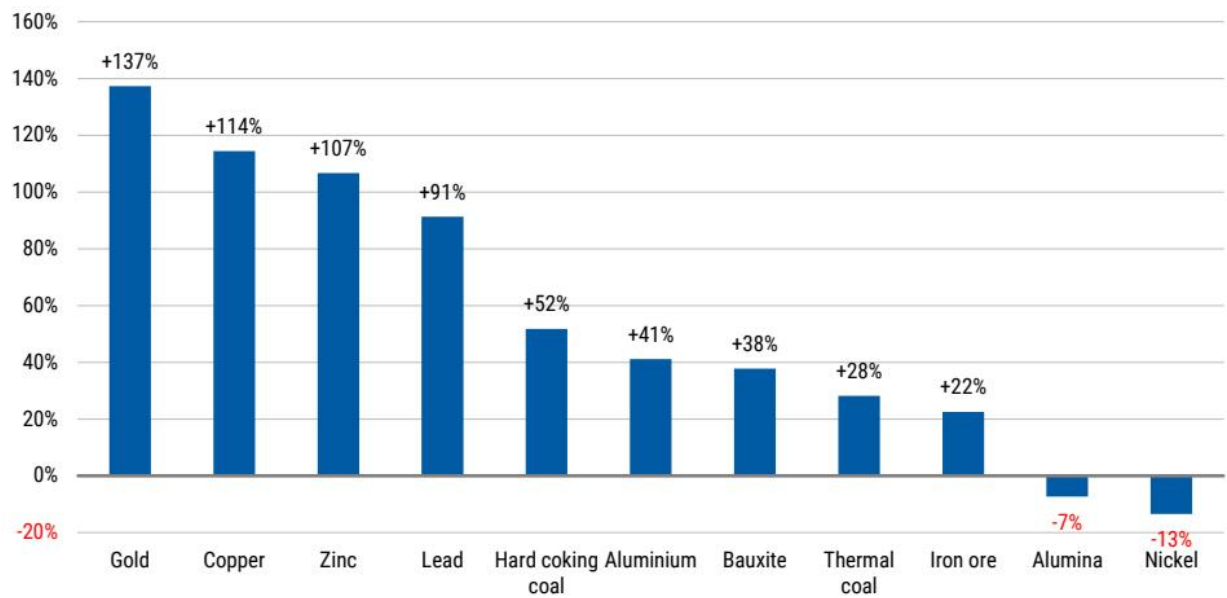
图表21：现货商品价格与边际生产成本对比
