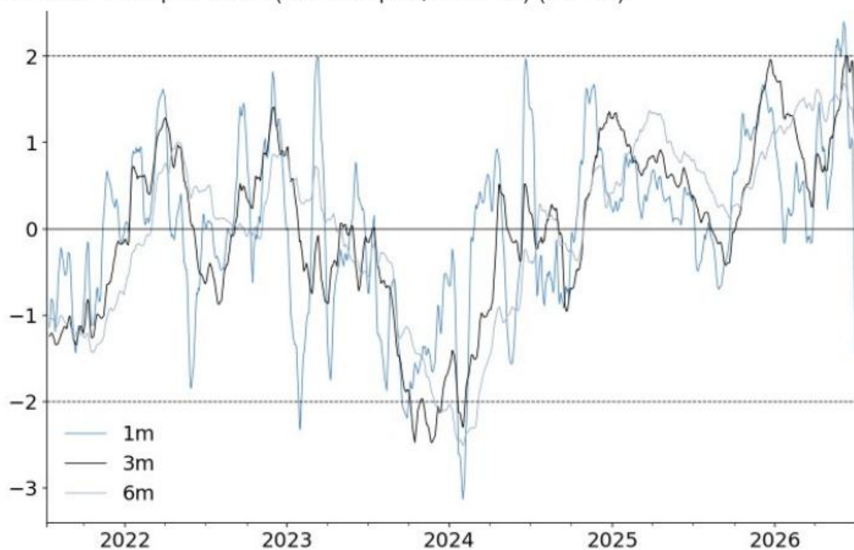
图表 9
